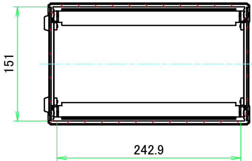
B-B ( 1 : 5 )
