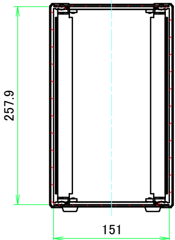
A-A ( 1 : 5 )
