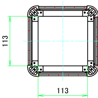
C-C ( 1 : 5 )
